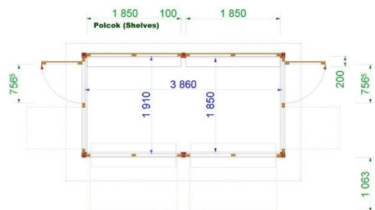
Alaprajz/layout
