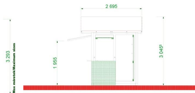
Oldalsó felületek Sides
